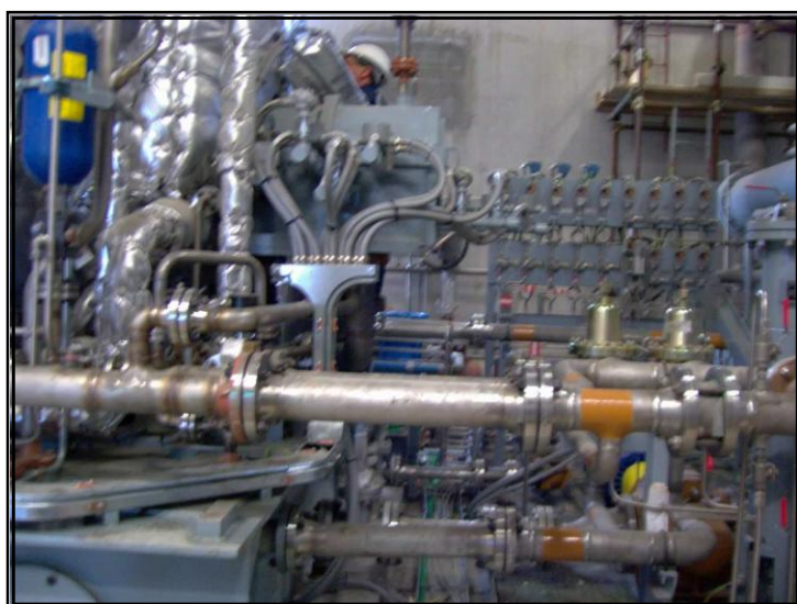
Collegamenti a skid centralina olio.
